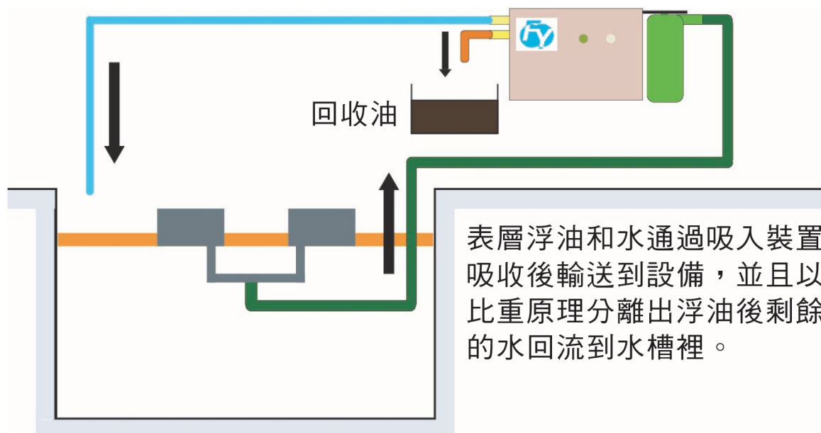
浮油回收機
